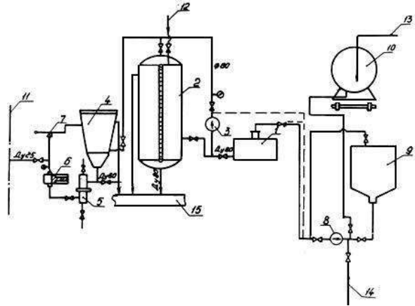
Рис. 2. Схема установки для дозирования силиката натрия.
