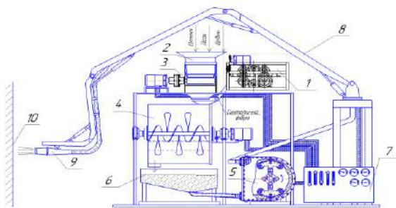
Рис. 7. Технологічний комплект малогабаритного обладнання для проведення торкрет-робіт в умовах будівельного майданчика: 1 - автомат-різчик фібри; 2 - дозувальний вузол; 3 - стрічковий живильник; 4 - бетонозмішувач гравітаційно-примусової дії; 5 - універсальний шланговий бетононасос; 6 - бункер з бетонною сумішшю; 7 - гідравлічна насосна станція; 8 - маніпулятор; 9 - торкрет-сопло з кільцевим насадком; 10 – поверхня, що торкретується.
