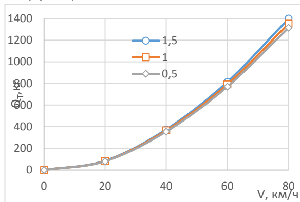
Рис. 2 - Зависимость сопротивления воздушной среды Q_T от скорости поезда с учетом конкретных значений коэффициентов местных сопротивлений
