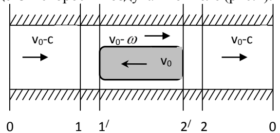
Рис.1. Скорости относительного движения в тоннеле
